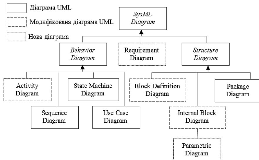
Рис. 1. SysML діаграми
