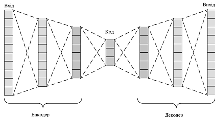
Рис. 4. Архітектура автоенкодера
