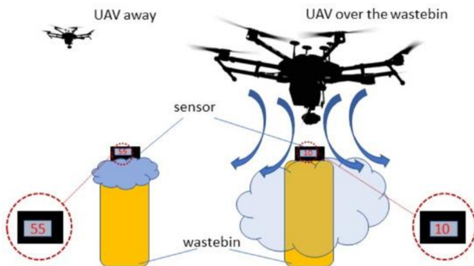
Рис. 3. Схематичне представлення експерименту з використанням БПЛА та датчика аміаку ChemDet, розміщеного на смітєвому баку, для демонстрації виникнення ефекту «змиву»
