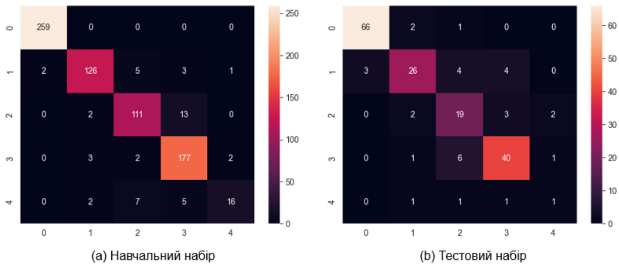
Рис. 2. Матриці плутанини для відображення точності навчання моделі ШНМ на даних UCI для: (a) навчального набору, (b) тестового набору
