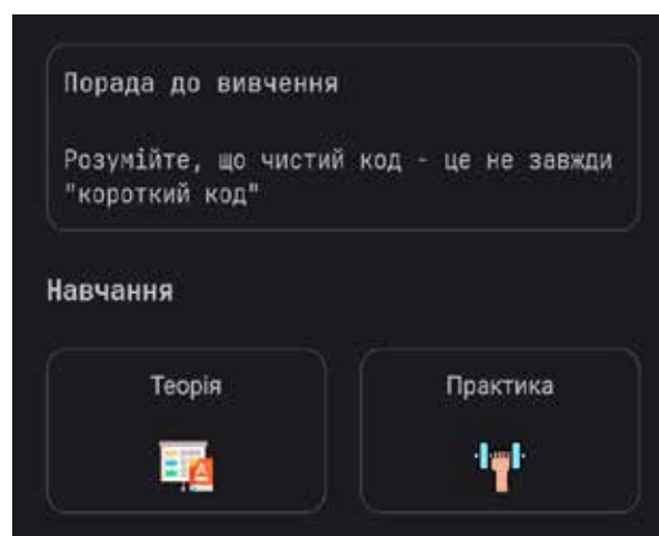
Рис. 3. Головний екран
