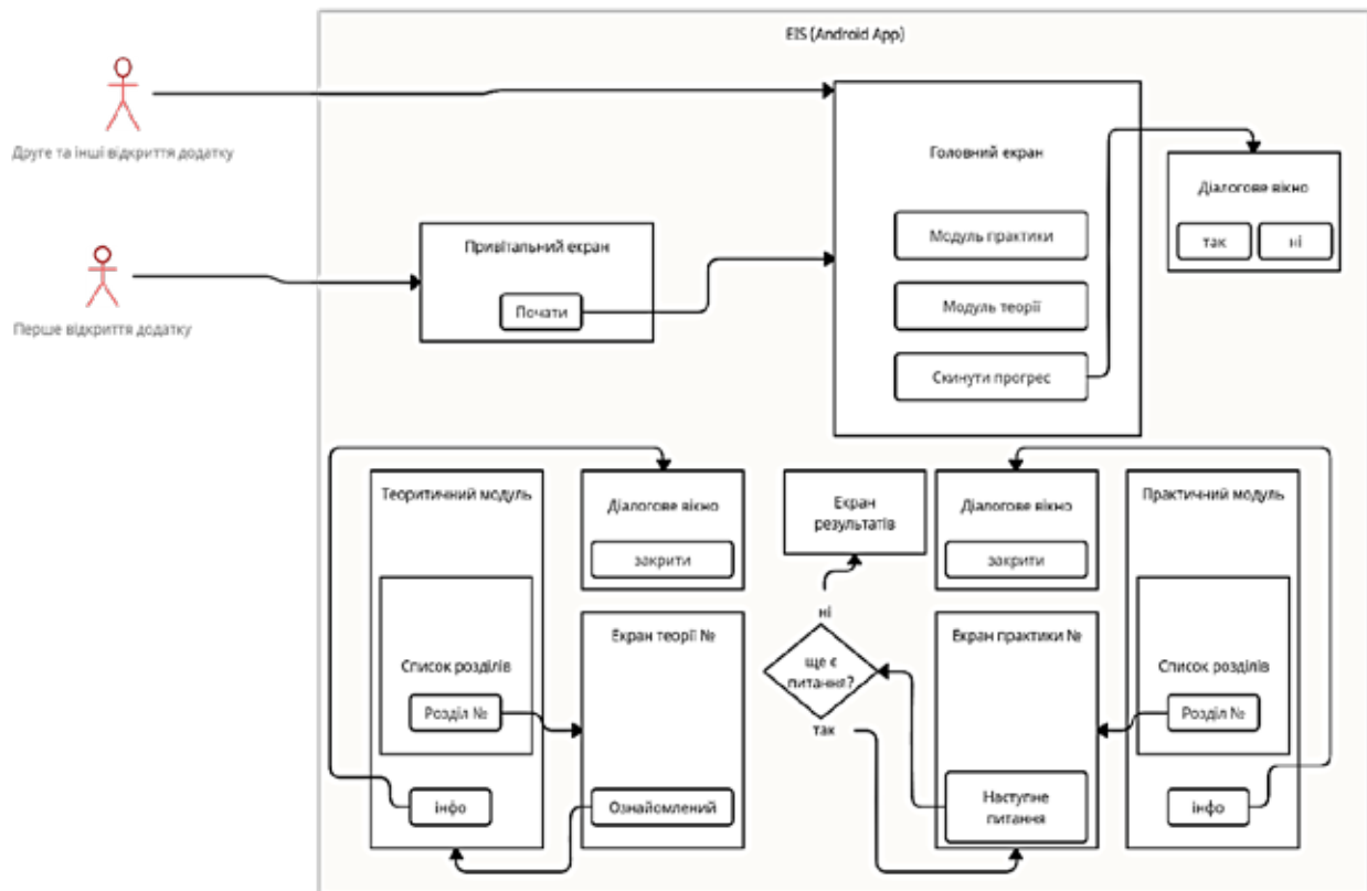
Рис. 2. Діаграма прецедентів
