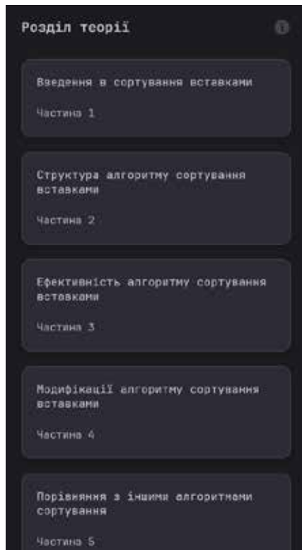
Рис. 7. Розділ Теорія
