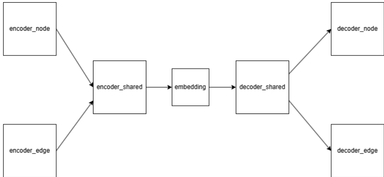
Рис. 1. Архітектура автоенкодера, що оброблює вершини та ребра електромережі
