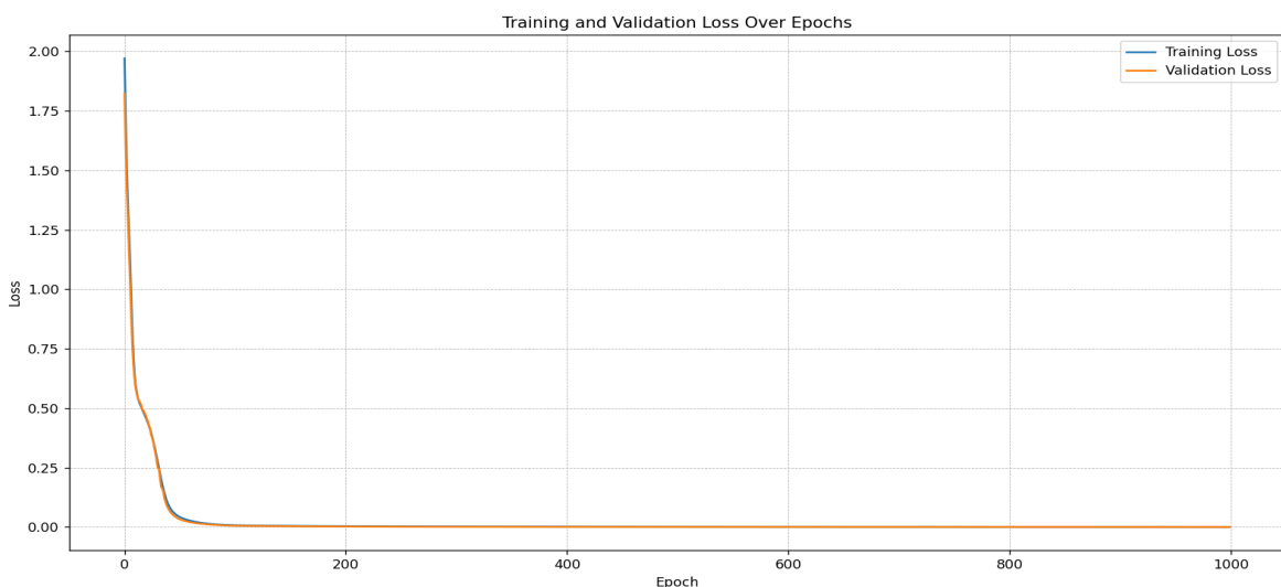
Рис. 4. Графік зміни помилки під час тренування моделі (Embedding Size = 45) на даних для тренування та валідації, використовуючи розроблений шар для графової мережі в енкодері
