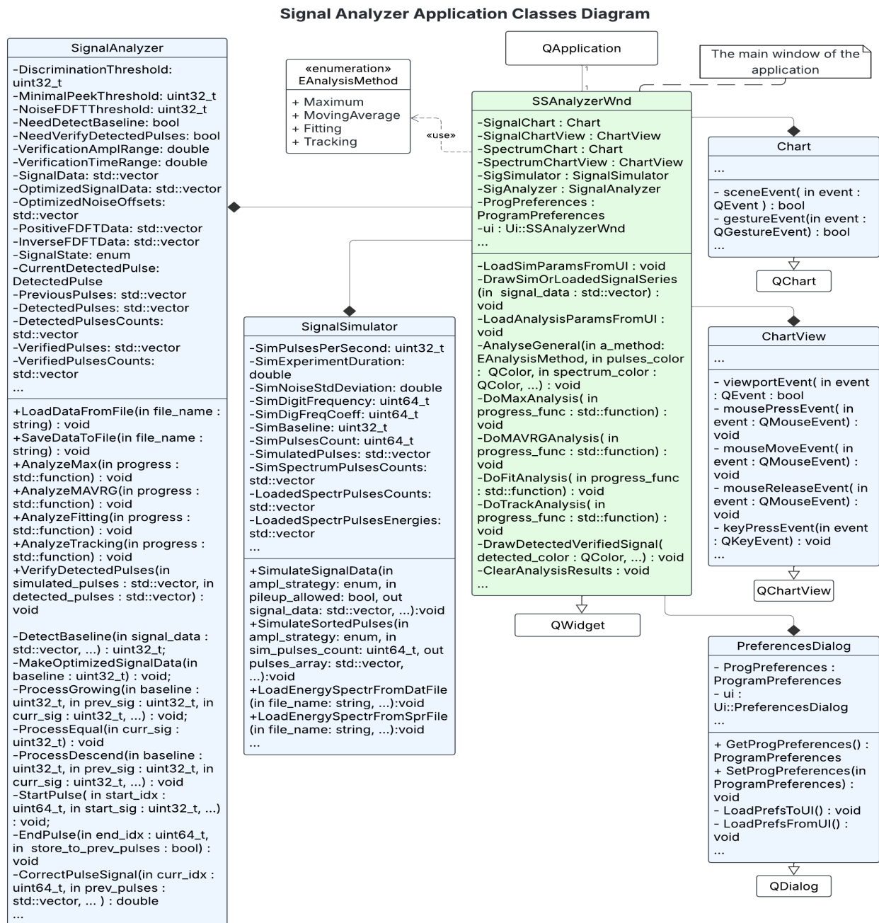
Рис. 3. UML діаграма класів, що реалізують функціонал додатку
