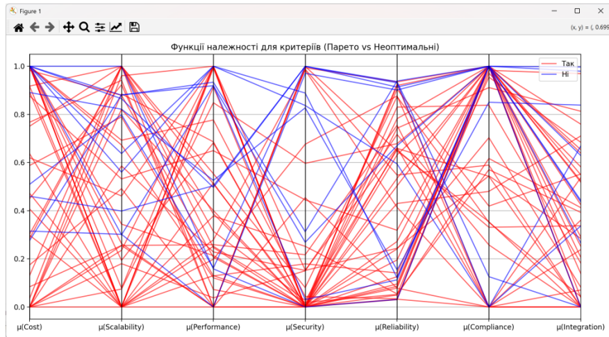
Рис. 2. Графіки «Функції належності для критеріїв (Парето vs Неоптимальні)»
