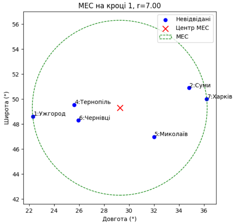
Рис. 1. Візуалізація використання мінімального охоплюючого кола для міст, що входять у нього при певному кроці обчислення на одному з вузлів
