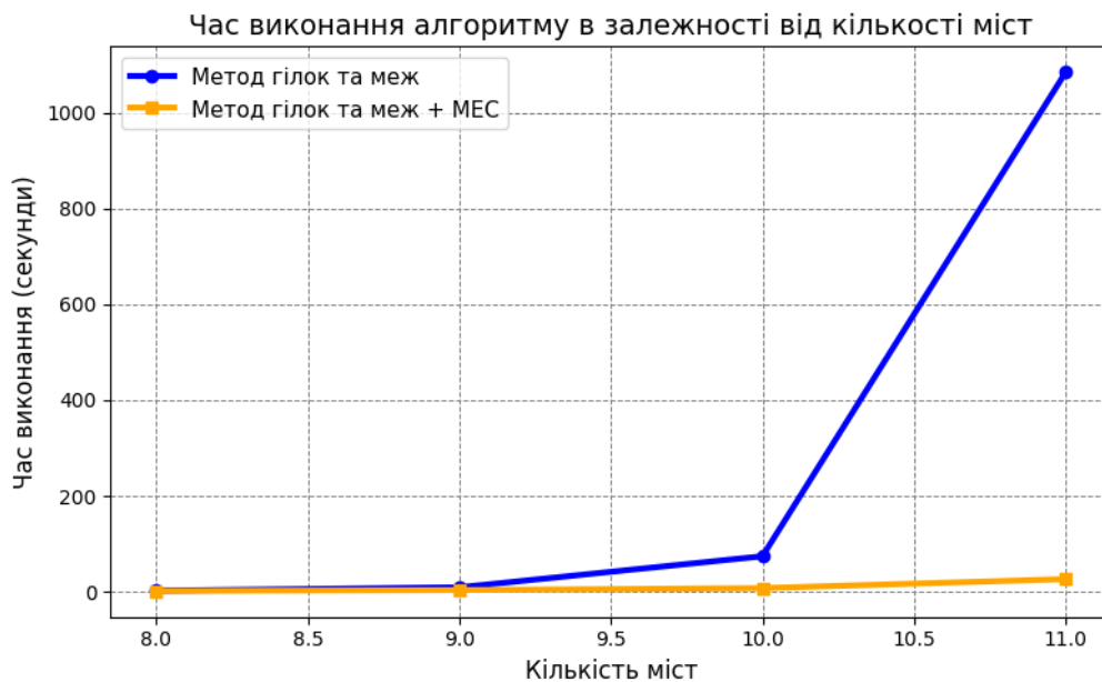
Рис. 3. Порівняльний графік залежності часу виконання від кількості міст методу гілок та меж без використання охоплюючого кола та з ним
