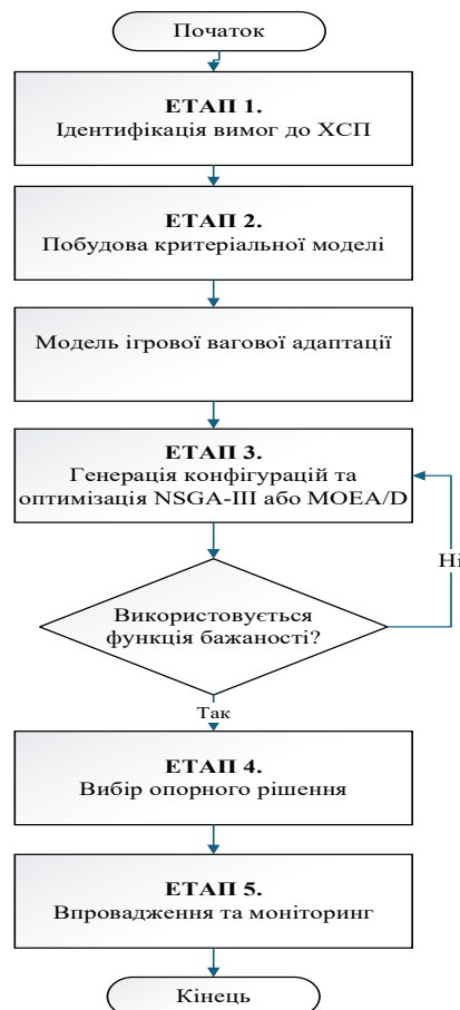
Рис. 1. Спрощена блок-схема алгоритму методу структурованого впровадження хмарної інфраструктури (CBXI)
