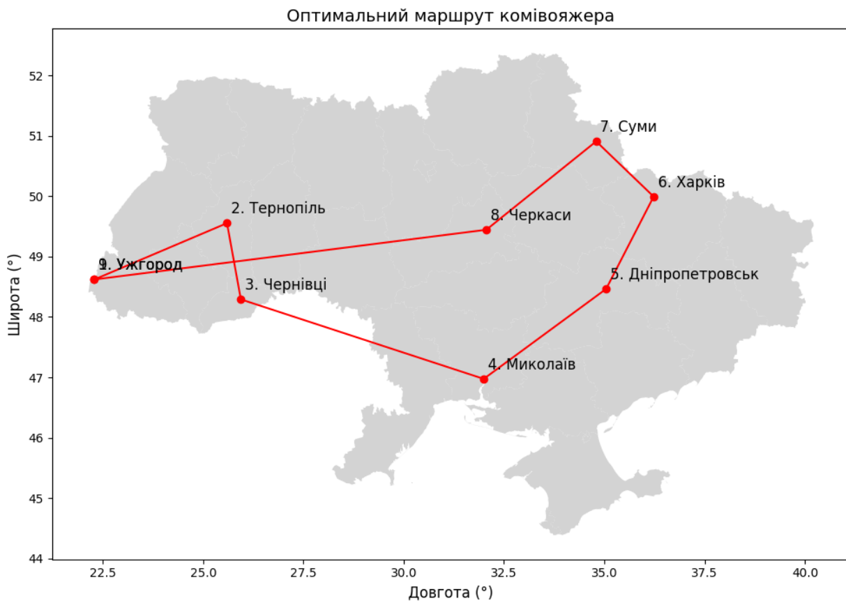
Рис. 2. Графічна візуалізація розв'язку задачі комівояжера для восьми міст України на основі методу гілок та меж із використанням мінімального охоплюючого кола
