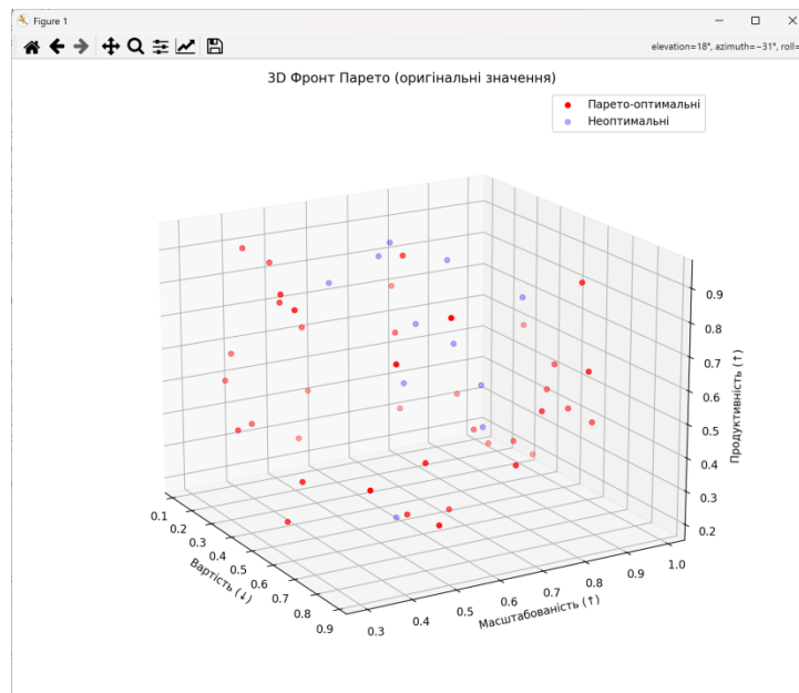
Рис. 3. 3D-візуалізація фронту Парето для задачі пошуку оптимальних ХС підприємства
