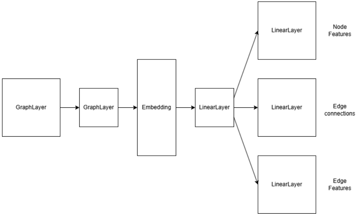
Рис. 3. Архітектура автоенкодера з шарами для обробки інформації про електромережу, яка визначена за допомогою графа
