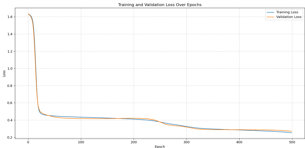
Рис. 2. Графік зміни помилки під час тренування моделі на даних для тренування та валідації (Embedding_Size=80)
