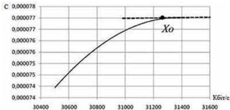
Рис. 7. Графік залежності часу затримки від навантаження каналу передавання
