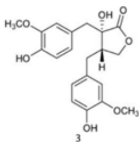
Рис. 7. 3-гідрокси-3,4-біс-(4-гідрокси-3-метоксибензил)-дигідрофуран-2-он
