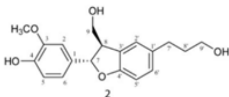
Рис. 6. 4-[3-гідроксиметил-5-(3-гідроксипропіл)-2,3-дигідробензофуран-2-іл]-2-метоксифенол
