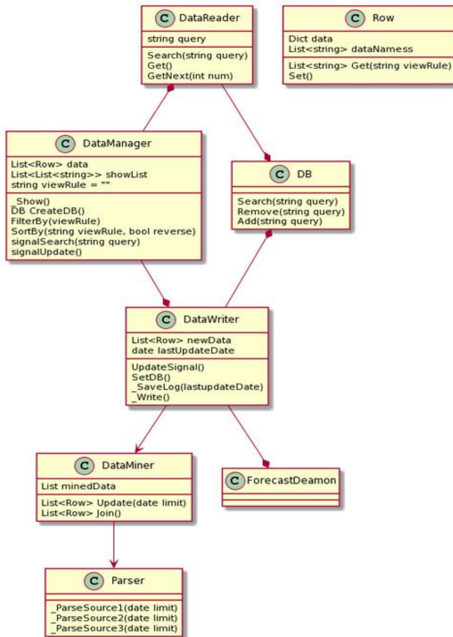
Рис. 2. Діаграма класів IC
