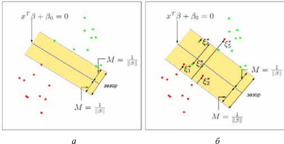
Рис. 3. Класифікатори з мінімальним зазором (а) і на опорних векторах (б)
