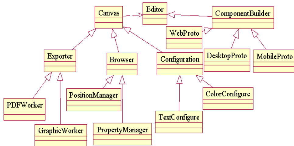
Рис. 3. Фрагмент діаграми класів системи
